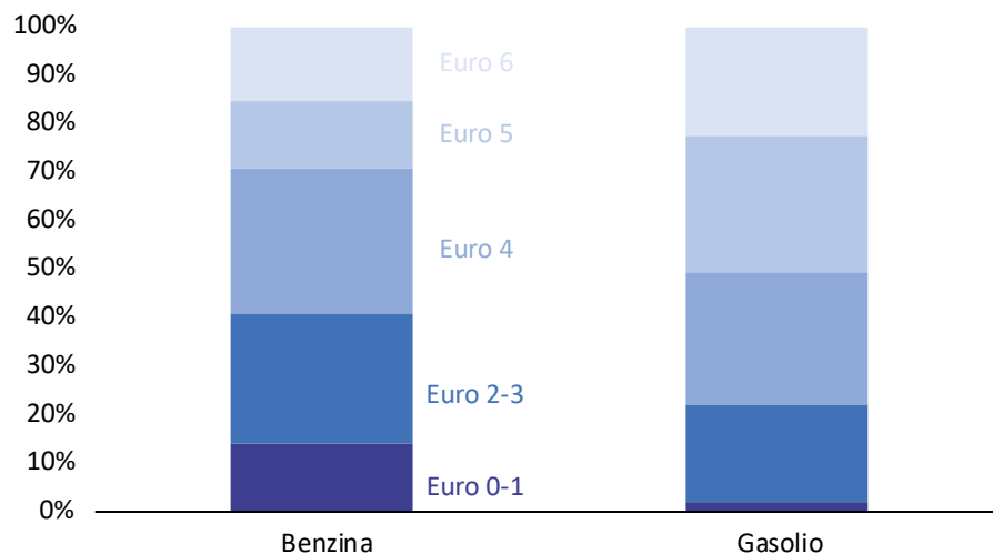
Distribuzione % degli autoveicoli a gasolio e benzina per standard di emissione. Veneto - Anno 2018
