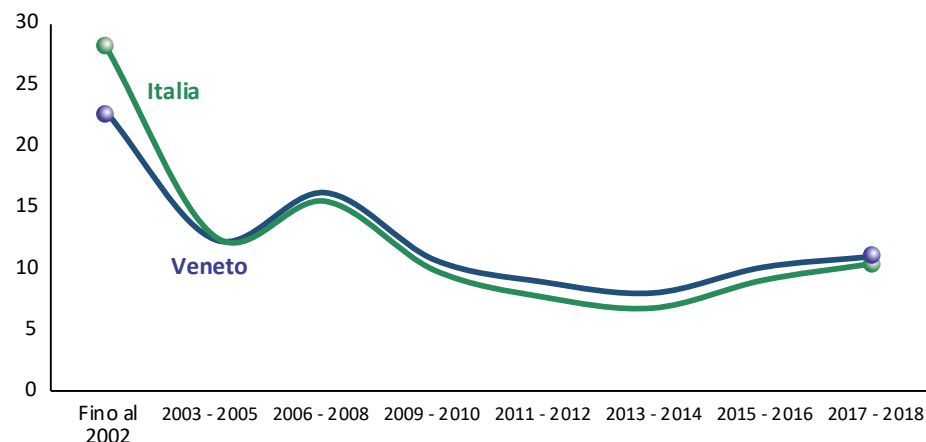
Distribuzione % degli autoveicoli per anno di immatricolazione. Veneto e Italia - Anno 2018
